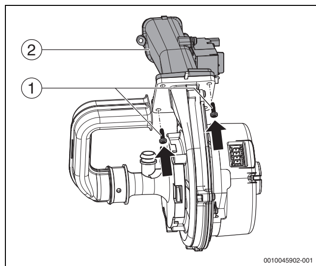
Fig. 87 Montaggio del tubo gas-aria, del ventilatore e della protezione antiriflusso
