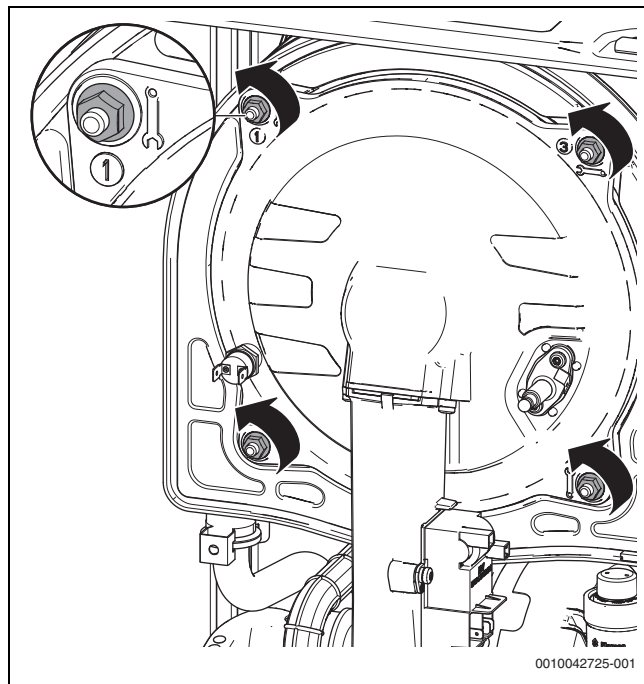
Fig. 46 Rimozione dei dadi di fissaggio
