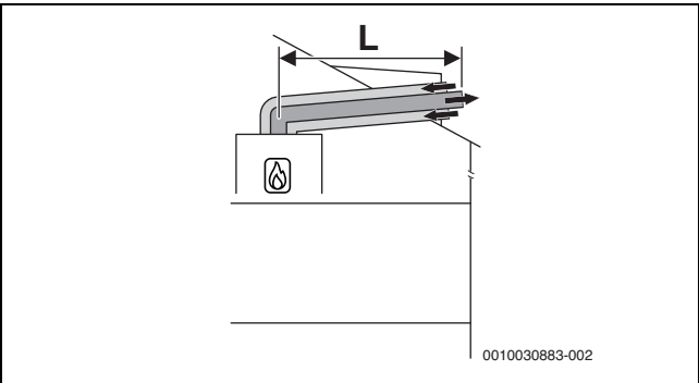
Fig. 8 Condotta di aspirazione aria comburente/evacuazione prodotti della combustione orizzontale concentrico secondo C 13x attraverso il tetto
