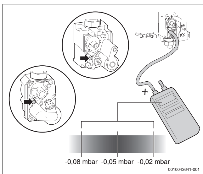
Fig. 40 Misurare la pressione differenziale
