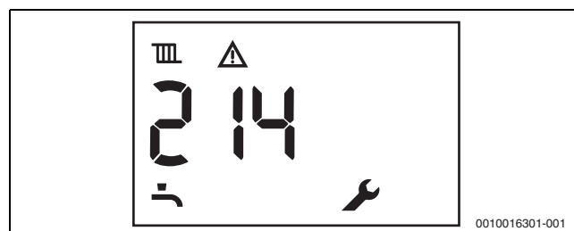
Fig. 156 Esempio: disfunzione non di blocco
