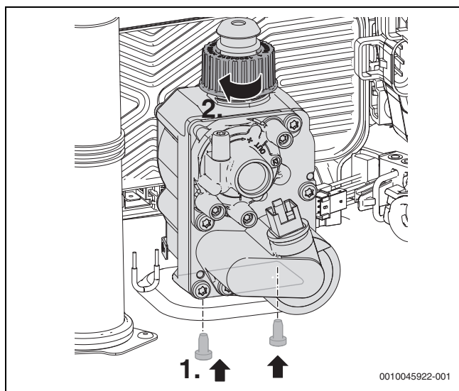
Fig. 96 Montaggio della vite e del dado
