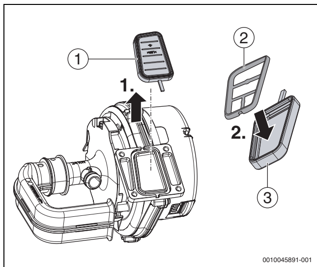
Fig. 85 Sostituzione della protezione antiriflusso
