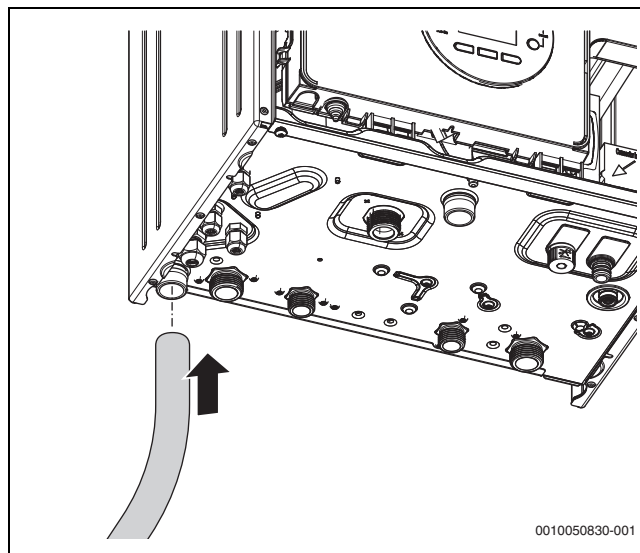
Fig. 27 Montaggio del tubo flessibile presso il sifone per la condensa
