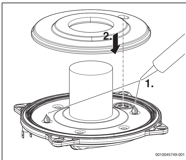
Fig. 69 Applicazione dell'adesivo silconico e installazione dell'isolamento nuovo
