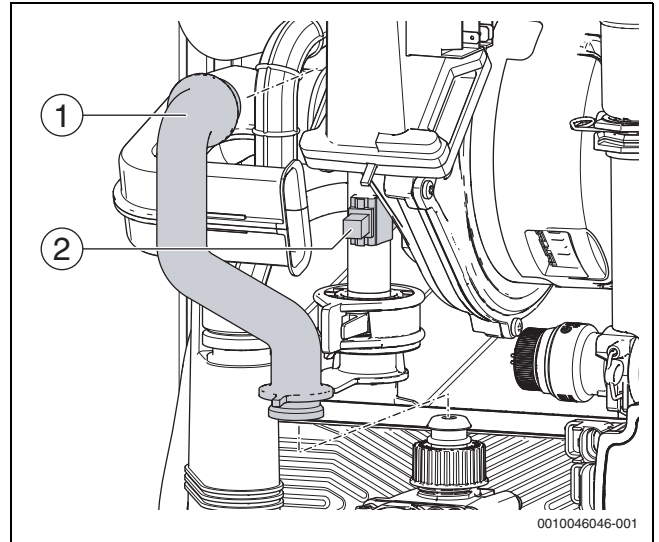
Fig. 135 Sostituzione della sonda NTC sul tubo di ritorno
