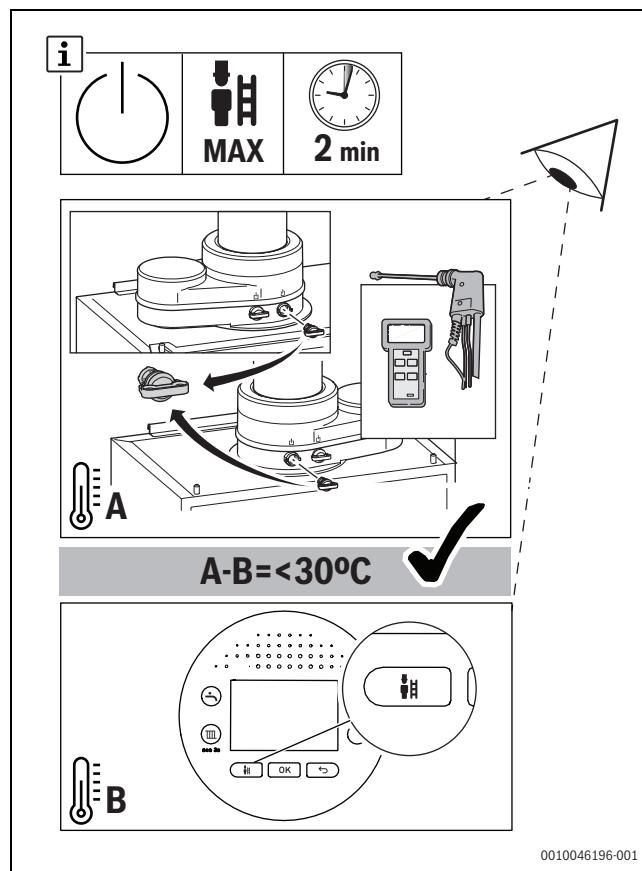
Fig. 78 Test di controllo dT
