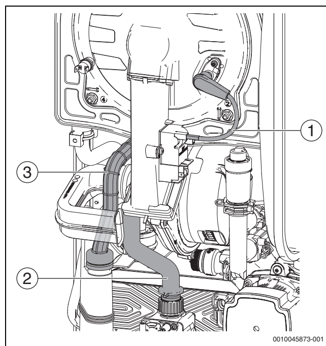
Fig. 79 Sportello bruciatore
