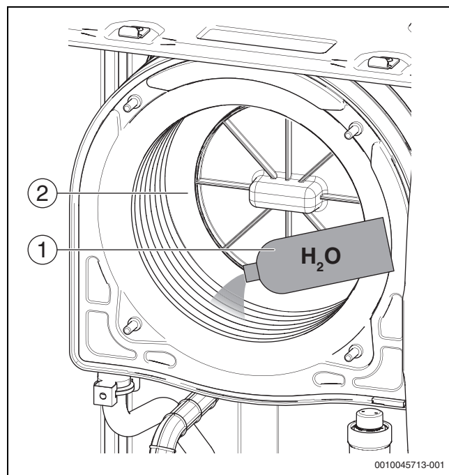
Fig. 52 Lavaggio con acqua
