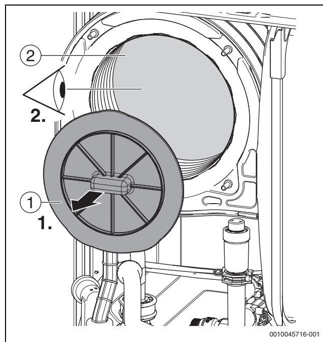
Fig. 53 Rimuovere la protezione dell'isolamento e controllare l'isolamento
