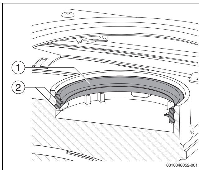
Fig. 137 Montaggio della guarnizione profilata
