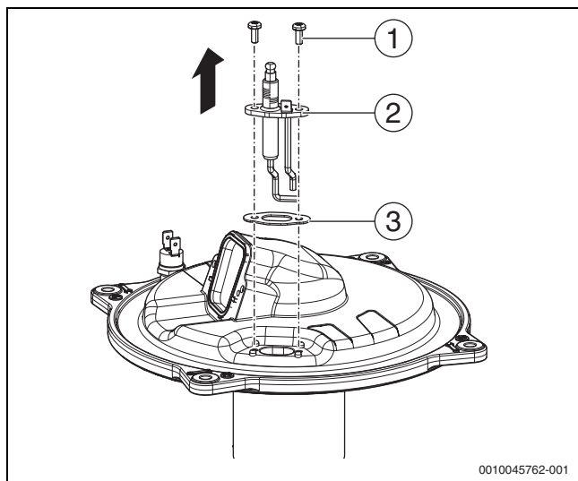
Fig. 70 Smontaggio dell'elettrodo accensione
