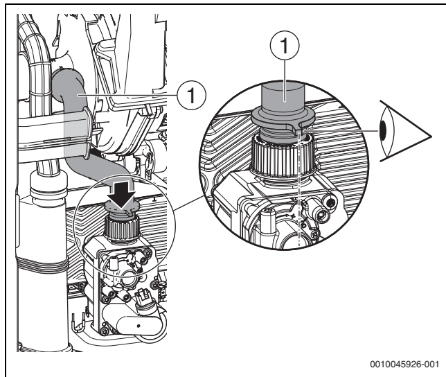
Fig. 126 Applicazione e allineamento del flessibile di collegamento gas
