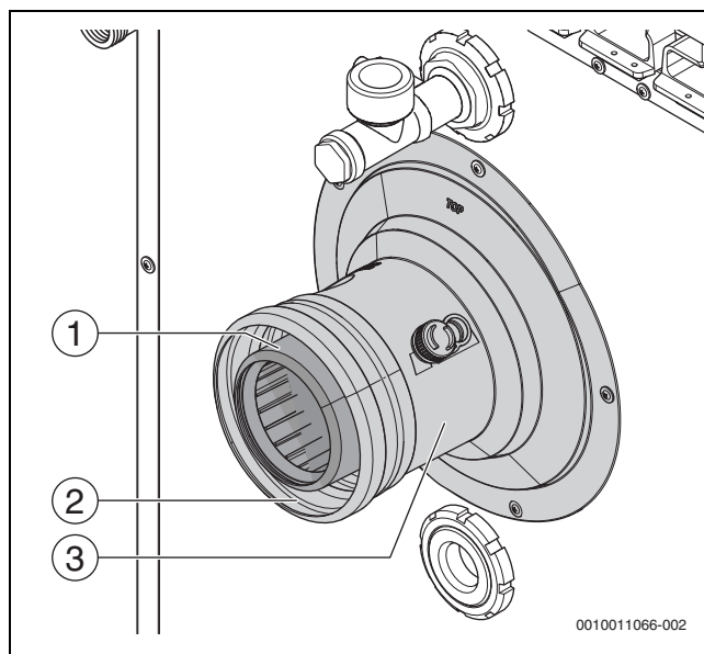
Fig. 18 Montaggio del collegamento di scarico dei gas combusti
