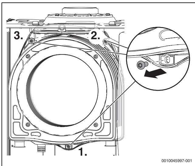
Fig. 105 Smontaggio dello scambiatore di calore
