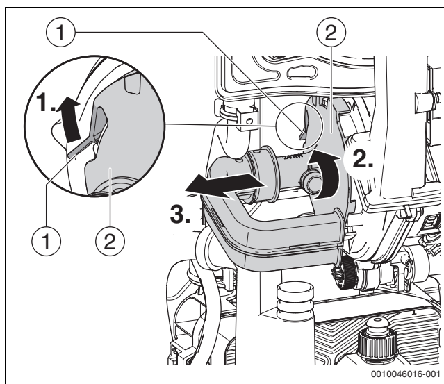
Fig. 114 Smontaggio del tubo Venturi
