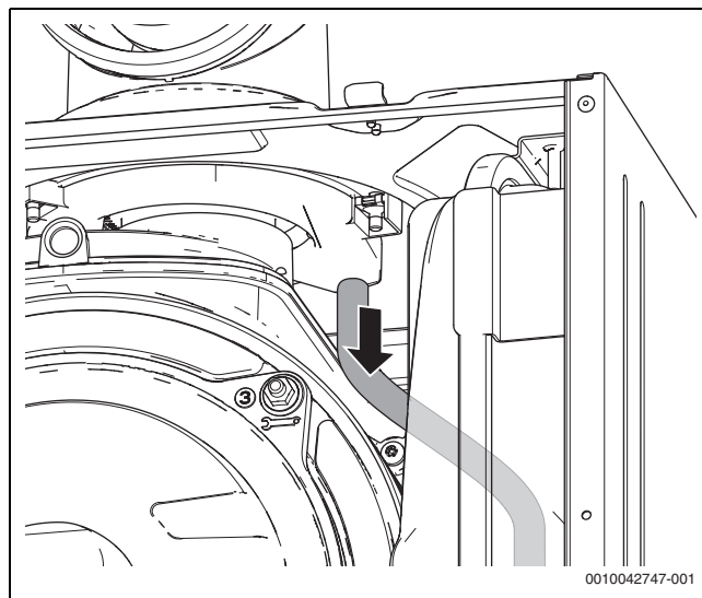
Fig. 148 Smontaggio della protezione contro la pioggia
