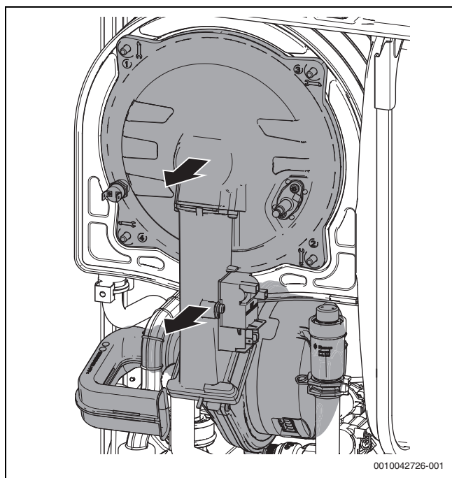
Fig. 47 Smontaggio dello sportello della camera di combustione
