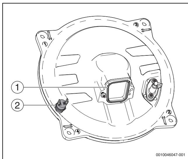
Fig. 128 Componenti del gruppo sportello della camera di combustione
