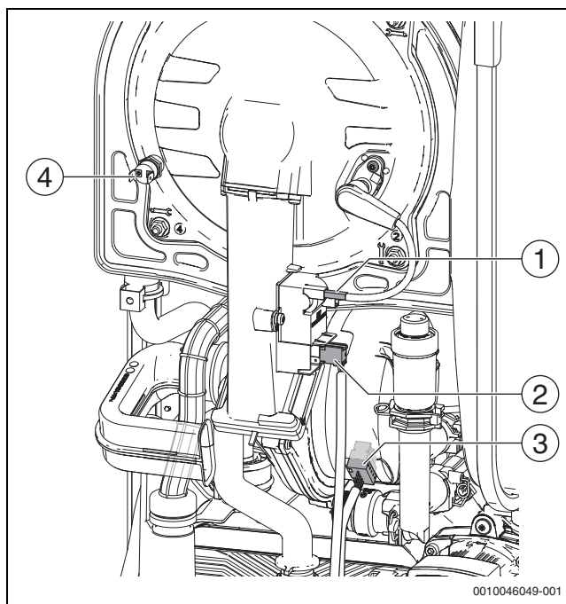
Fig. 130 Collegamento del cavo
