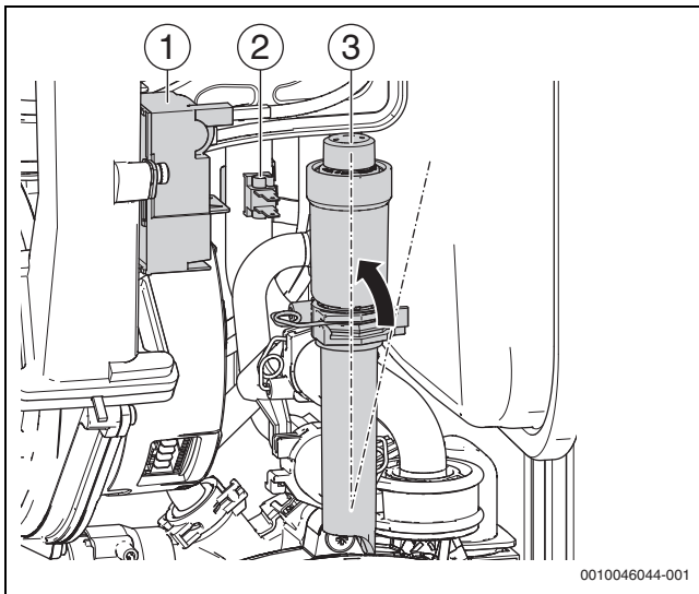
Fig. 133 Montaggio della sonda NTC nuova sul tubo di ritorno
