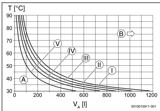
Fig. 25 Curve caratteristiche del vaso d'espansione
