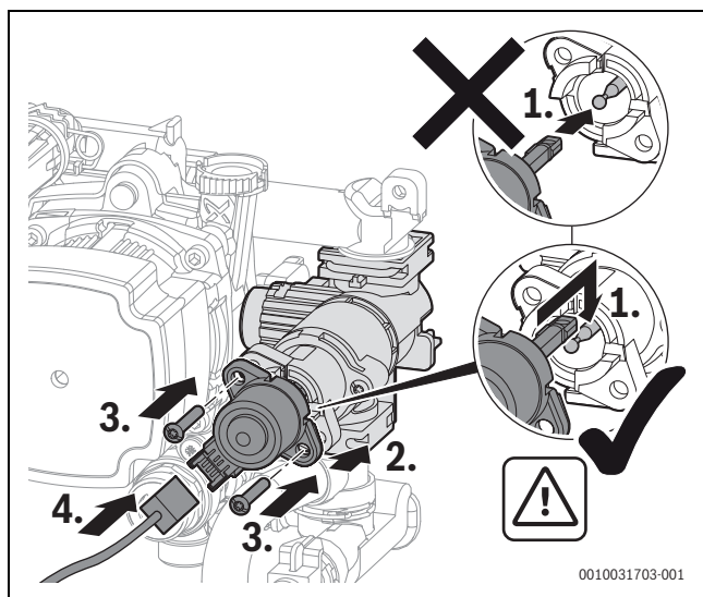
Fig. 154 Montaggio del motorino dalla valvola a 3 vie
