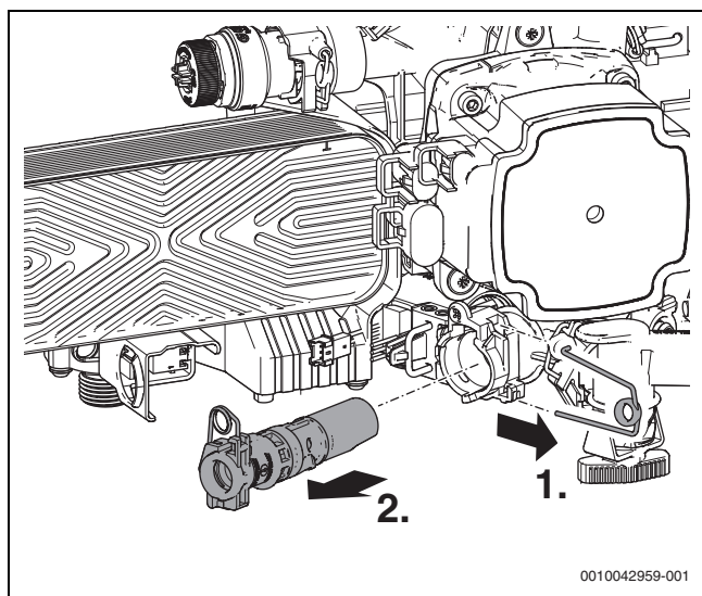
Fig. 143 Sostituzione del silenziatore
