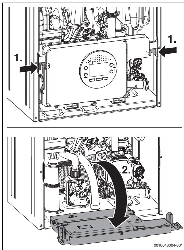
Fig. 32 Ribaltare verso il basso la scheda elettronica
