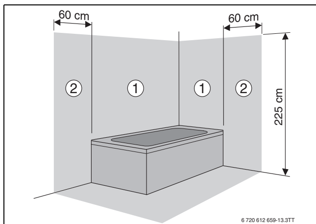
Fig. 29 Zone di sicurezza
