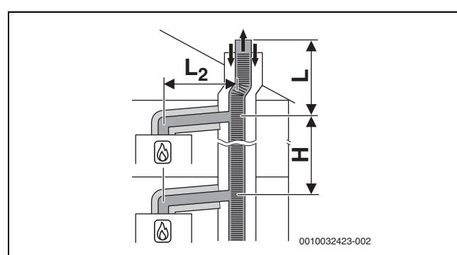
Fig. 23 Collettore scarico combusto secondo C_{(14)3x} con condotto di evacuazione prodotti della combustione collettivo e condotto di aspirazione aria comburente/evacuazione prodotti della combustione concentrico nel luogo di posa
