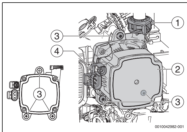
Fig. 155 Smontare il circolatore di riscaldamento
