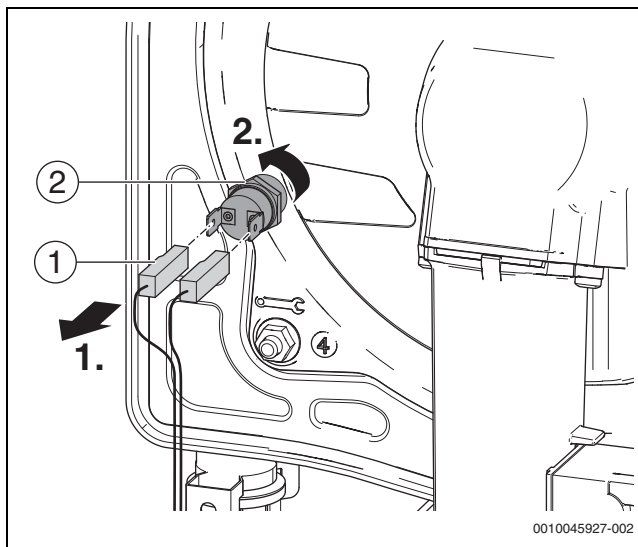
Fig. 98 Smontaggio del limitatore temperatura di sicurezza a riarmo
