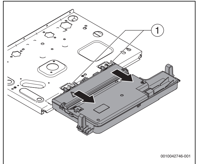
Fig. 140 Sostituire l'unità di servizio
