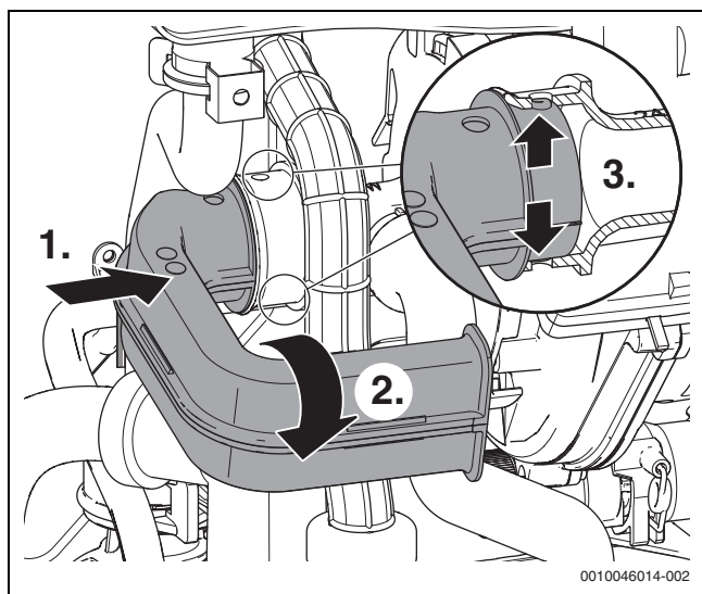
Fig. 112 Montaggio del tubo di immissione aria nuovo
