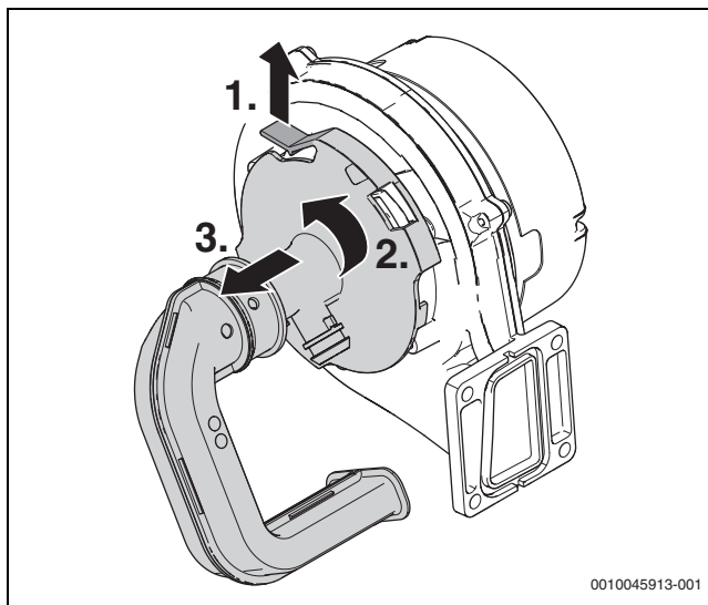
Fig. 91 Smontaggio del ventilatore
