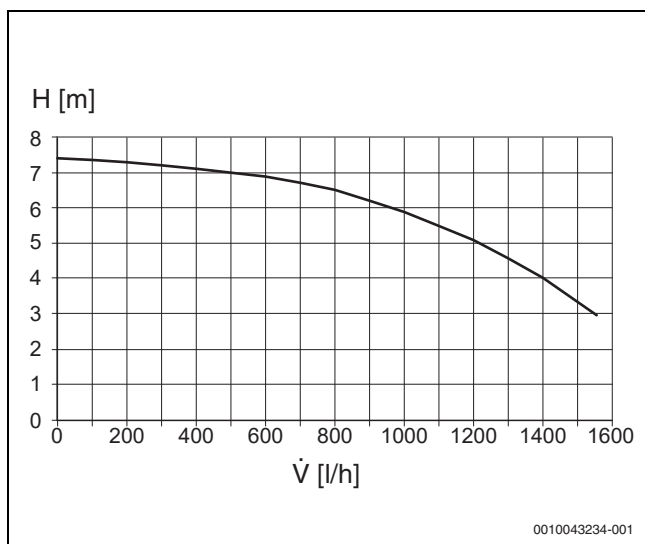
Fig. 35 Curva caratteristica del circolatore di riscaldamento (velocità costante)
