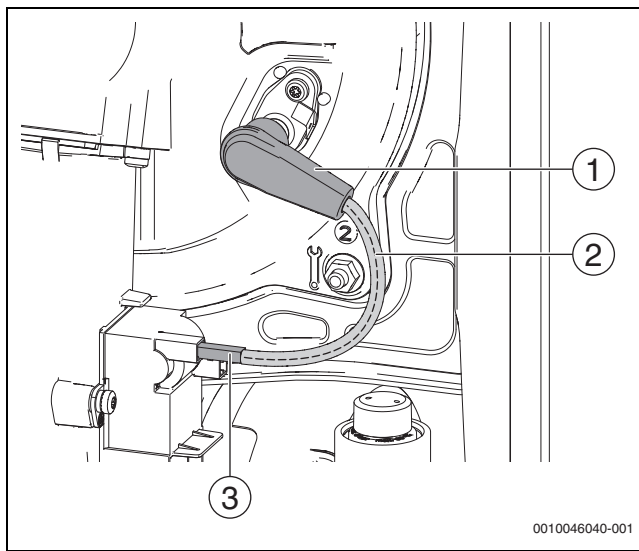
Fig. 131 Sostituzione del cavo elettrodo d'accensione
