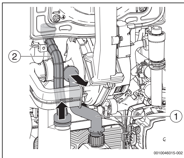
Fig. 113 Smontaggio del tubo flessibile condensa e del flessibile di collegamento gas
