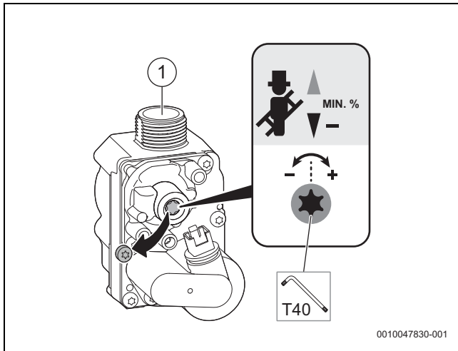
Fig. 59 Regolare il tenore di CO 2 (valvola SIT in alto, valvole Honeywell in basso)
