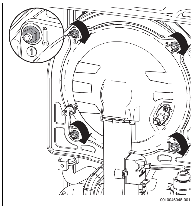
Fig. 129 Applicare lo sportello della camera di combustione sullo scambiatore di calore
