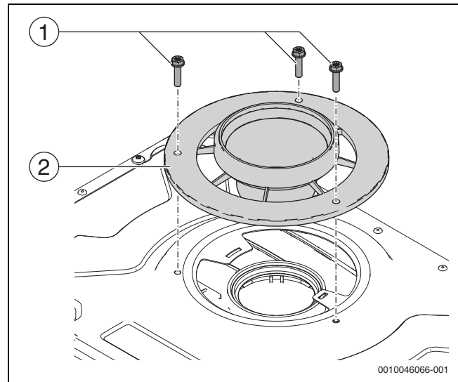
Fig. 61 Smontaggio del set condotto di evacuazione prodotti della combustione e dell'adattatore per condotto gas combusti
