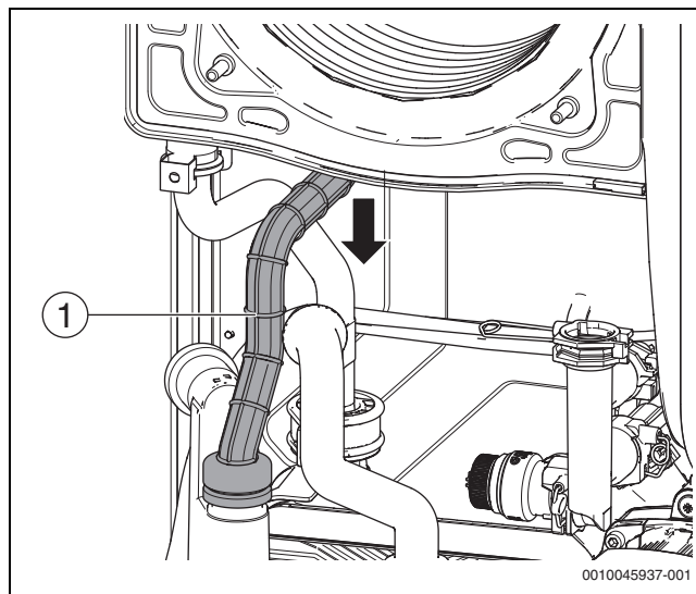
Fig. 102 Distacco del tubo flessibile per scarico condensa
