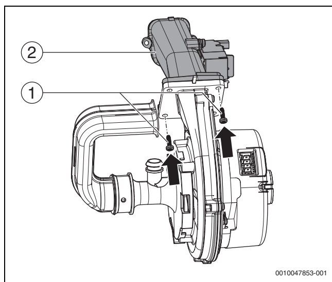
Fig. 120 Montaggio del tubo gas-aria
