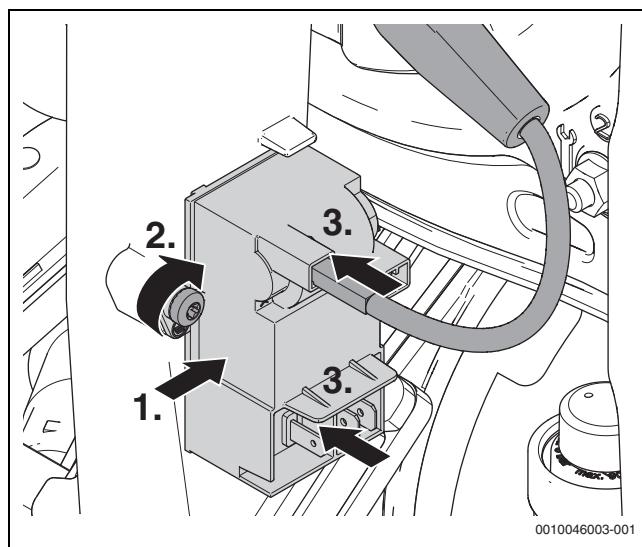
Fig. 110 Montaggio del trasformatore d'accensione nuovo
