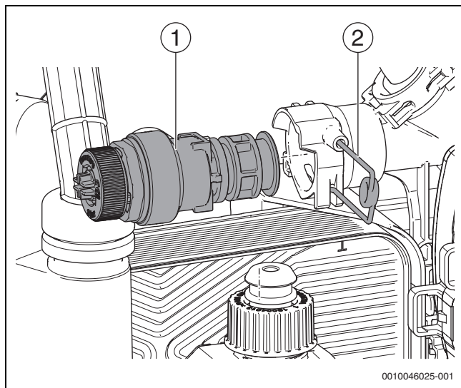
Fig. 146 Smontaggio della valvola di sicurezza
