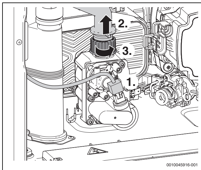
Fig. 93 Smontaggio del flessibile di collegamento gas, del giunto ad innesto e del dado
