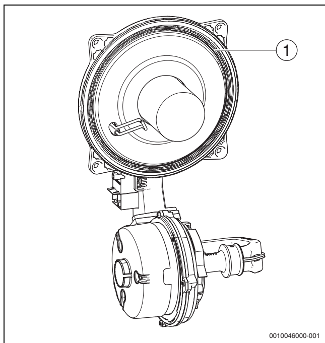
Fig. 108 Montaggio della guarnizione profilata nuova
