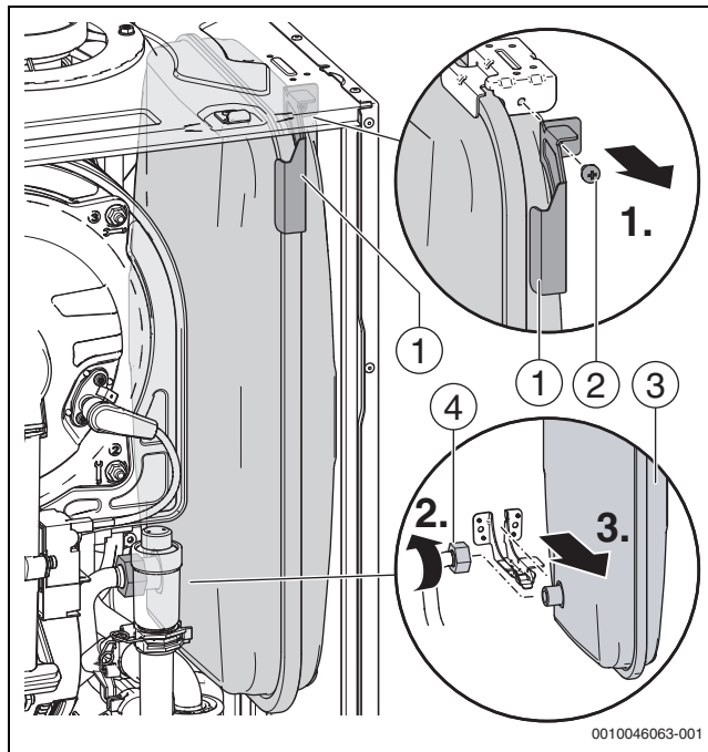
Fig. 138 Smontaggio del vaso d'espansione
