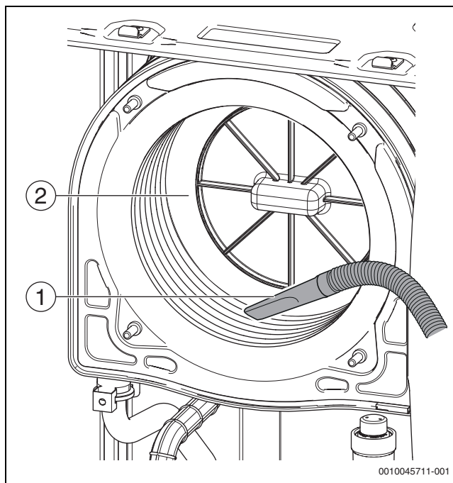
Fig. 50 Operazione di aspirazione
