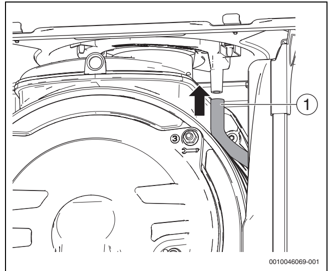
Fig. 65 Montaggio del tubo flessibile di scarico acqua
