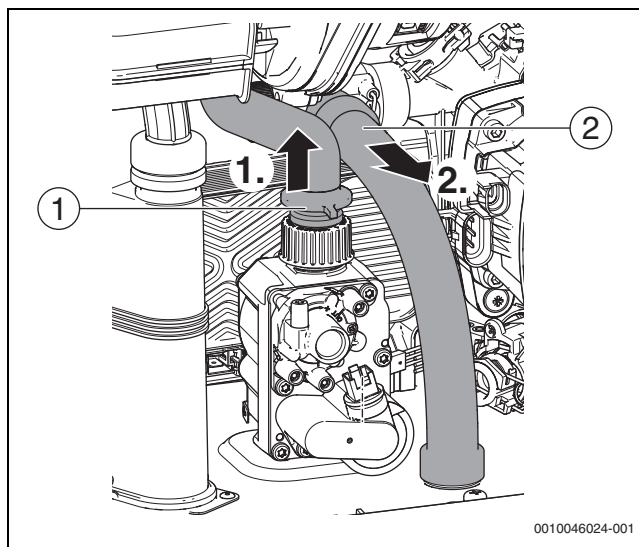
Fig. 145 Distacco del flessibile di collegamento gas e del tubo flessibile di scarico
