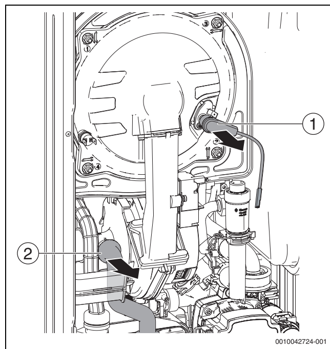
Fig. 45 Scollegare il cavo elettrodo d'accensione del set di elettrodi e staccare il flessibile di collegamento gas
