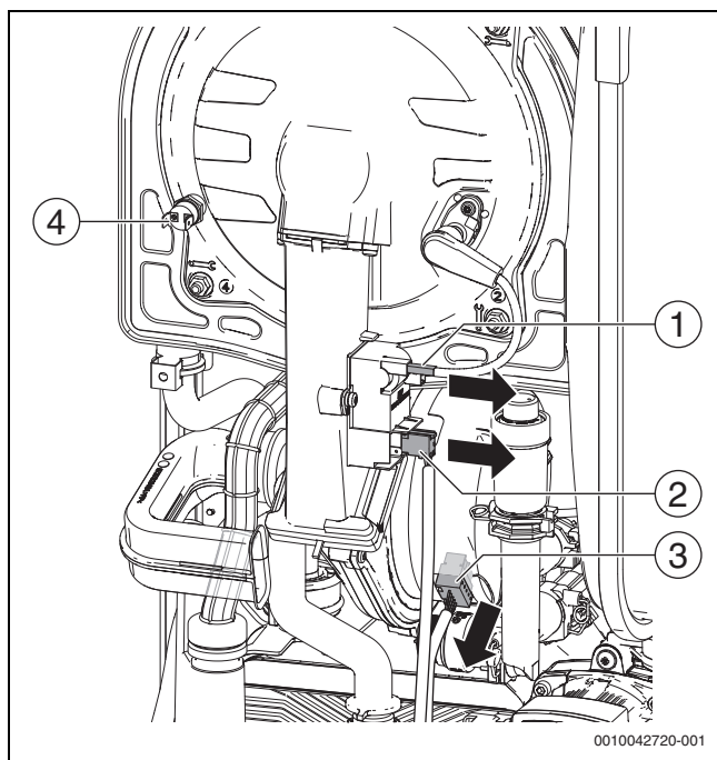
Fig. 44 Scollegamento della connessione elettrica
