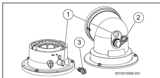
Fig. 38 Punto di misurazione per la prova di tenuta ermetica del condotto del sistema di aspirazione aria/evacuazione dei prodotti della combustione
