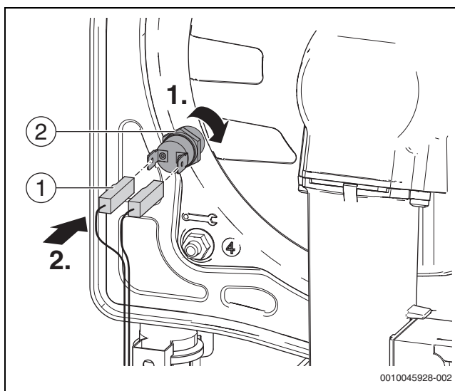
Fig. 99 Montaggio del limitatore temperatura di sicurezza a riarmo
