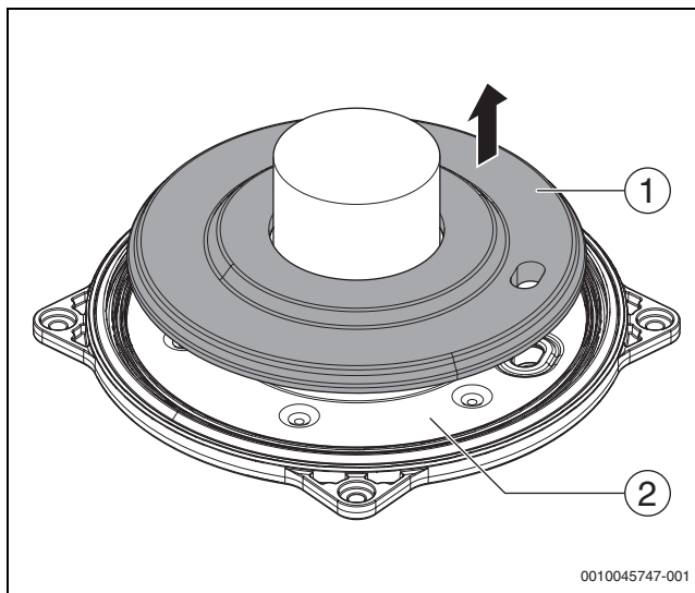
Fig. 68 Smontaggio dell'isolamento
