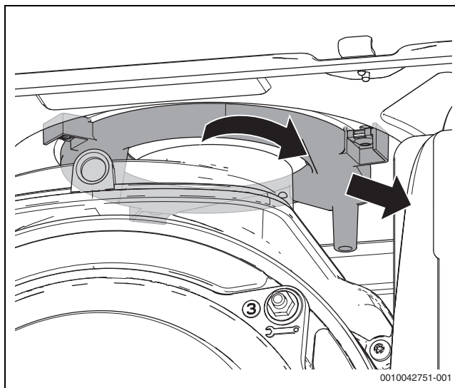
Fig. 152 Smontaggio della protezione contro la pioggia
