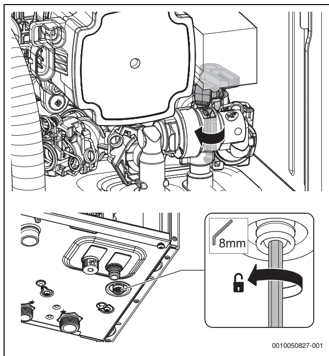
Fig. 67 Valvola di scarico
