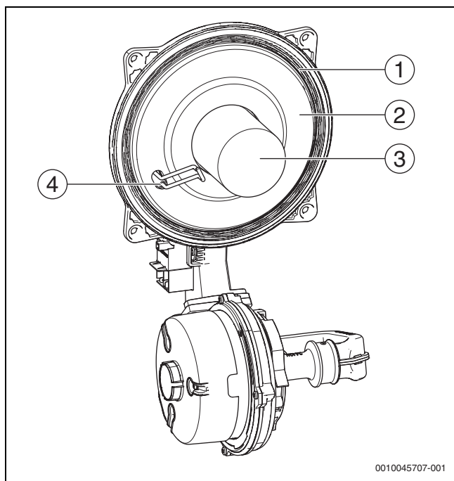
Fig. 48 Gruppo sportello della camera di combustione
