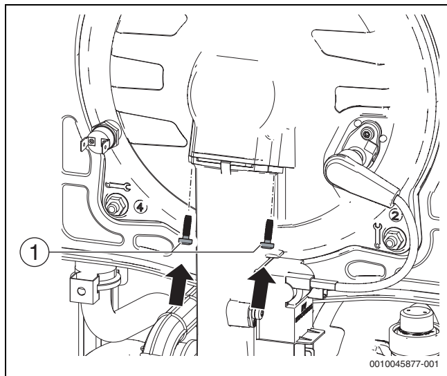
Fig. 88 Montaggio del tubo gas-aria sullo sportello della camera di combustione
