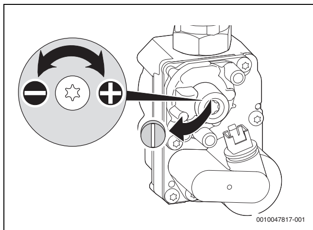
Fig. 41 Rimozione del piombino sulla vite di regolazione
