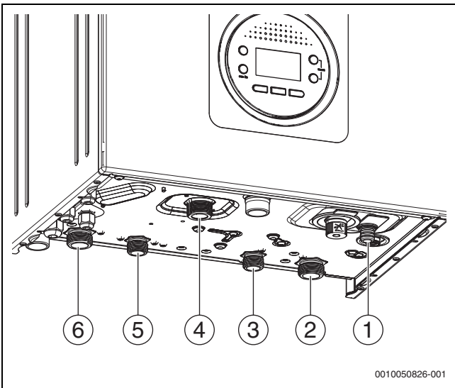
Fig. 28 Collegamenti lato gas e lato acqua (accessori)
