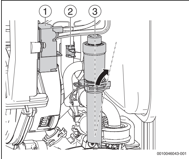
Fig. 132 Smontaggio della sonda NTC sul tubo di ritorno
