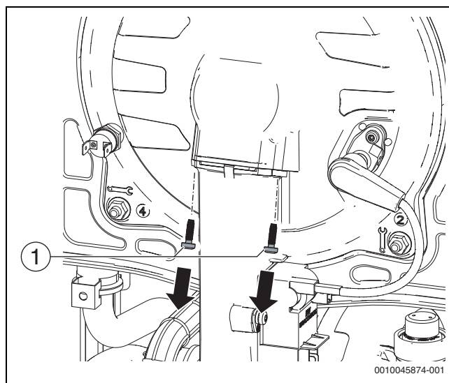
Fig. 118 Smontaggio delle viti
