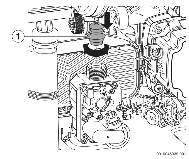
Fig. 125 Applicazione del diaframma nuovo e del dado del gas
