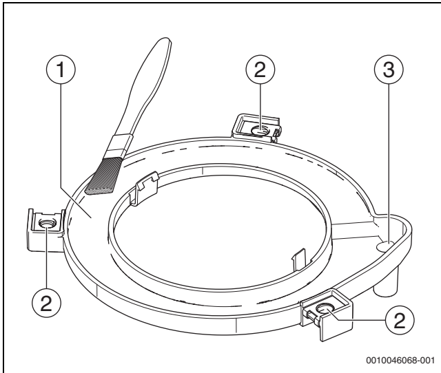
Fig. 63 Pulizia del parapioggia
