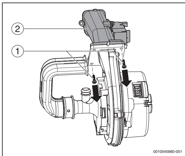
Fig. 84 Smontaggio del tubo gas-aria
