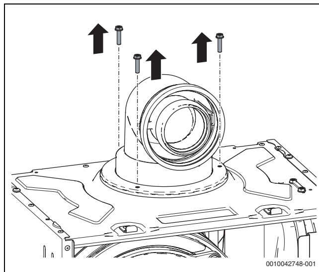
Fig. 149 Rimozione delle viti di fissaggio
