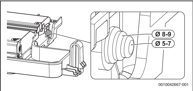
Fig. 34 Passacavo
