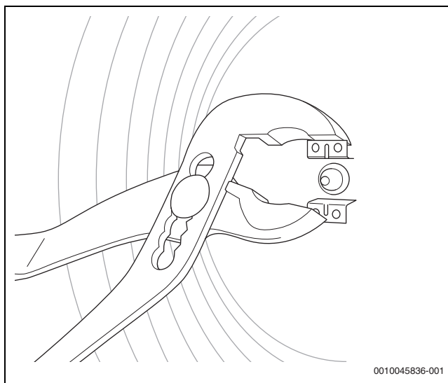
Fig. 75 Rimozione dell'inserto centrale
