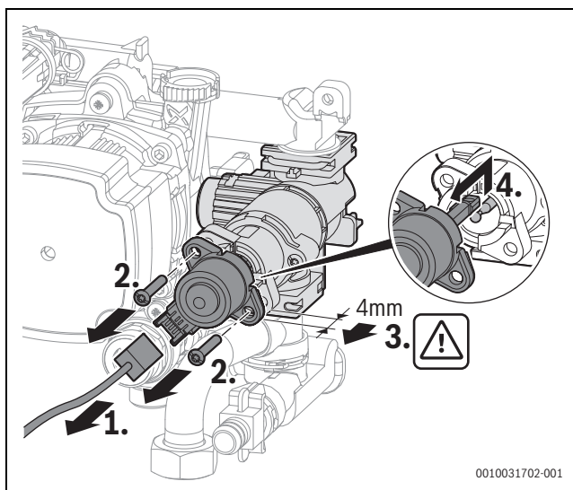
Fig. 153 Smontaggio del motorino dalla valvola a 3 vie
