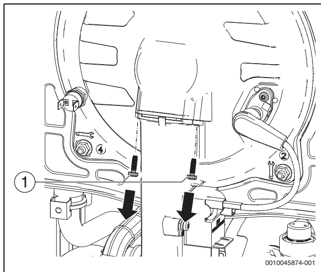
Fig. 80 Smontaggio delle viti
