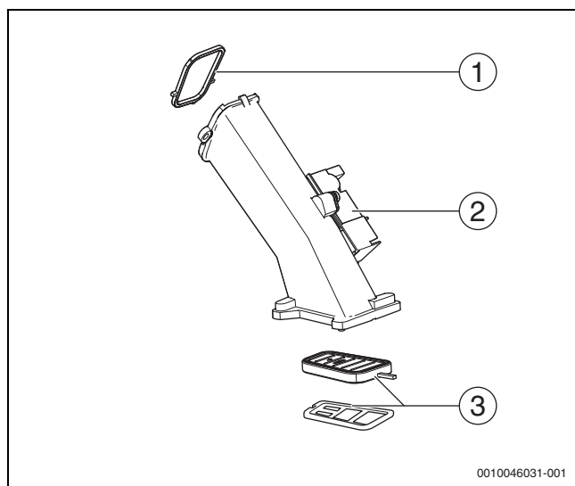
Fig. 119 Componenti del tubo gas-aria
