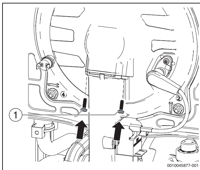
Fig. 83 Montaggio delle viti nello sportello della camera di combustione
