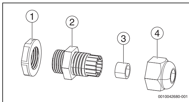
Fig. 31 Componenti del pressacavo a vite
