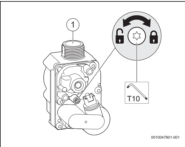
Fig. 37 Controllo della pressione di ingresso del gas
