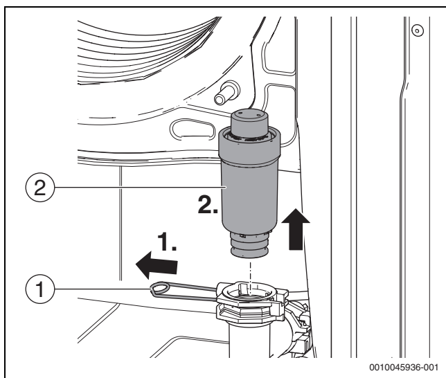
Fig. 101 Smontare il disaeratore automatico
