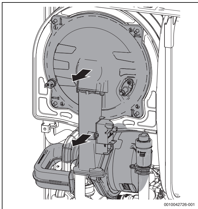
Fig. 100 Smontaggio del gruppo sportello della camera di combustione
