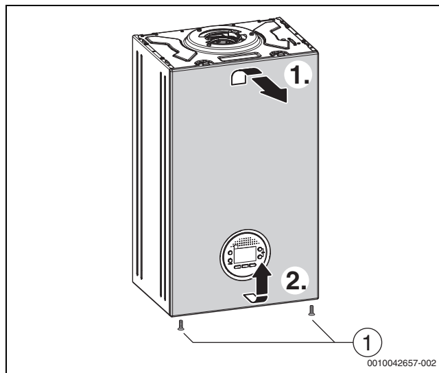
Fig. 26 Rimozione del rivestimento anteriore
