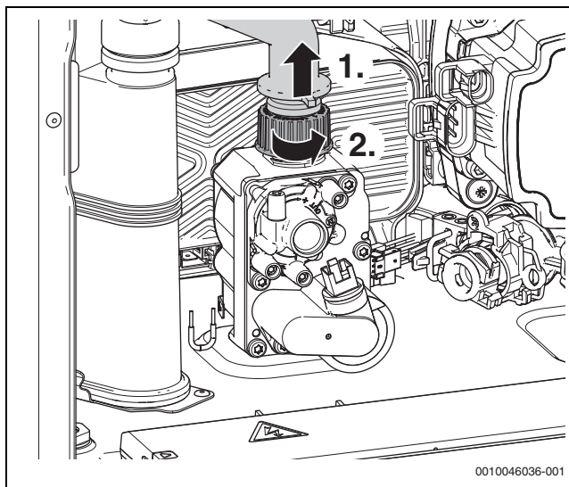
Fig. 122 Smontaggio del flessibile di collegamento gas e del dado del gas
