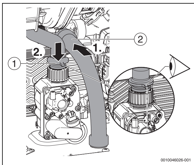
Fig. 147 Montaggio del flessibile di collegamento gas e del tubo flessibile di scarico
