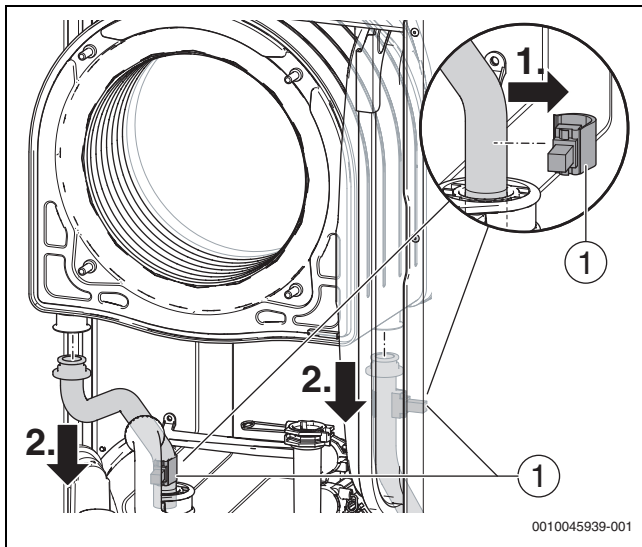
Fig. 104 Smontaggio delle sonde NTC e dei tubi
