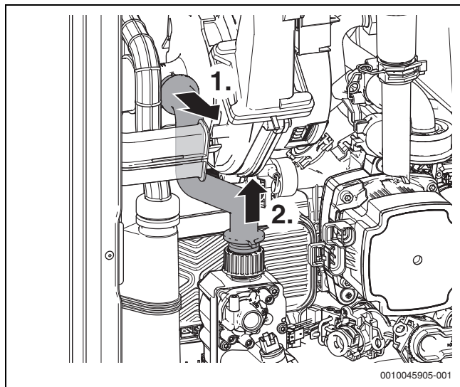
Fig. 89 Smontaggio del flessibile di collegamento gas
