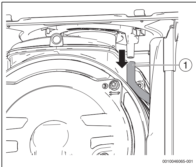
Fig. 60 Smontaggio del tubo flessibile di scarico acqua
