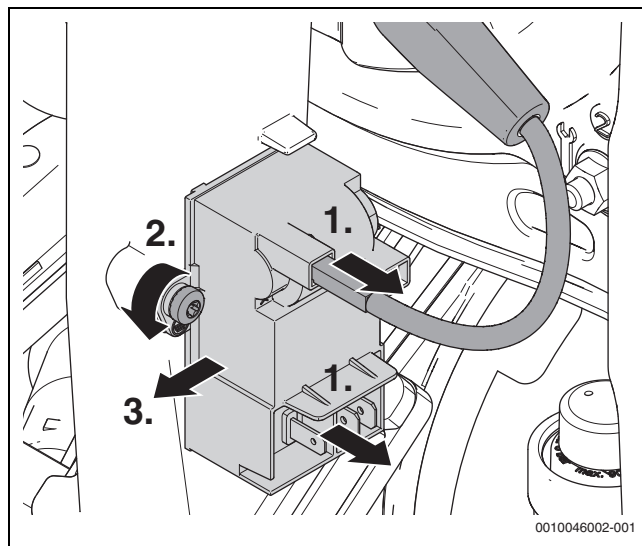
Fig. 109 Smontaggio del trasformatore d'accensione
