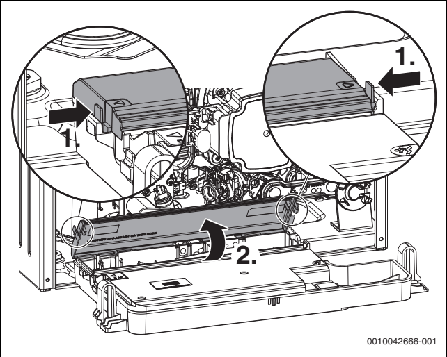
Fig. 33 Apertura del pannello protettivo di servizio
