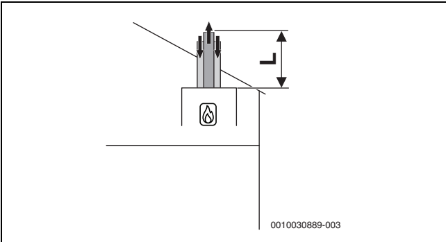
Fig. 10 Condotta di aspirazione aria comburente/evacuazione prodotti della combustione verticale concentrico secondo C 33x
