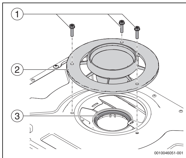
Fig. 136 Smontaggio dell'adattatore per condotto gas combusti e del set condotto di evacuazione prodotti della combustione
