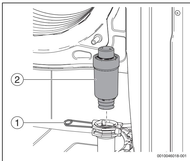
Fig. 142 Sostituzione del disaeratore automatico
