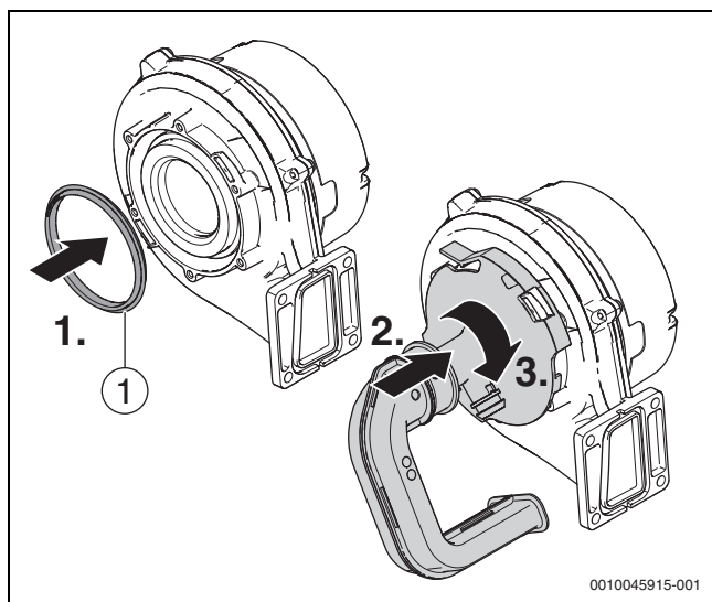
Fig. 92 Montaggio del ventilatore
