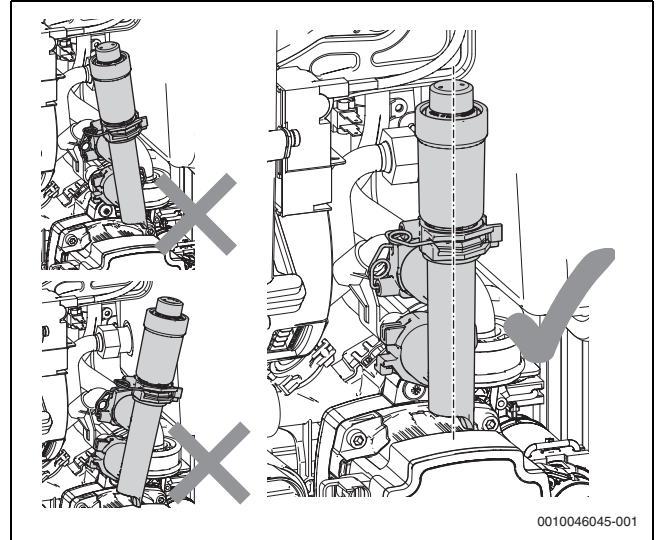
Fig. 134 Posizione del disaeratore
