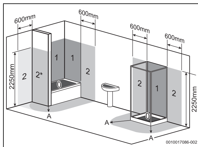
Fig. 24 Zone di sicurezza (esempio)
