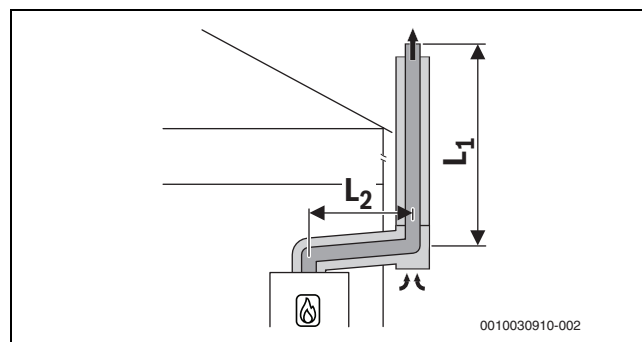
Fig. 15 Condotta di aspirazione aria comburente/evacuazione prodotti della combustione concentrico secondo C_{53x} sulla parete esterna
