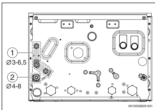
Fig. 30 Diametro cavo
