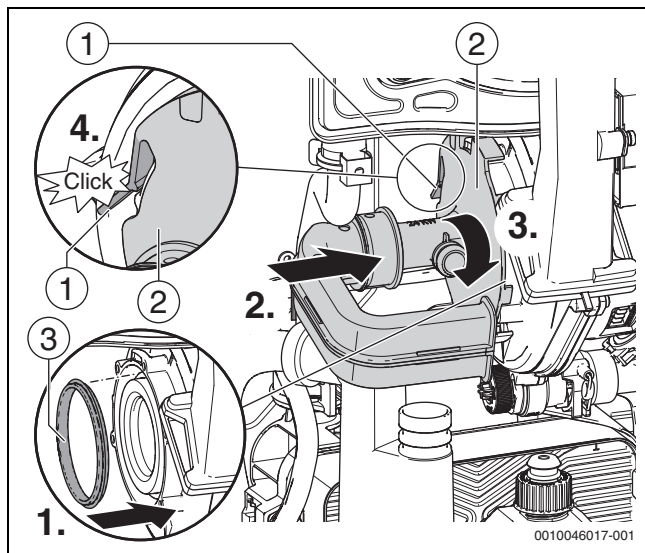
Fig. 115 Montaggio del tubo Venturi nuovo
