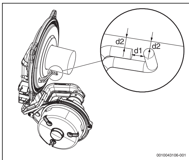
Fig. 57 Verifica dell'elettrodo di controllo e di accensione
