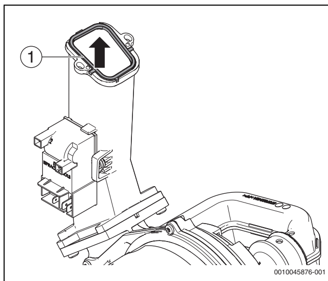
Fig. 82 Smontaggio della guarnizione
