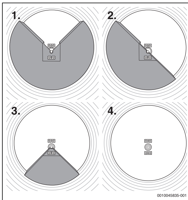
Fig. 74 Fasi di smontaggio dell'isolamento
