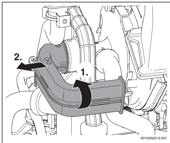
Fig. 111 Smontaggio del tubo di immissione aria
