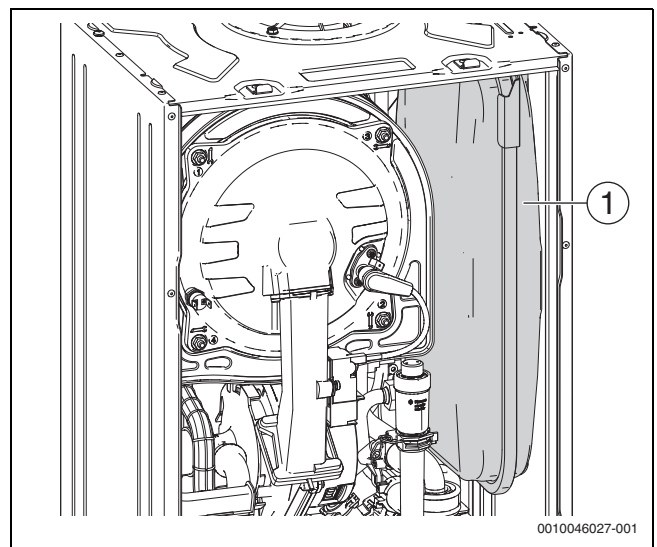
Fig. 66 Controllo del vaso d'espansione
