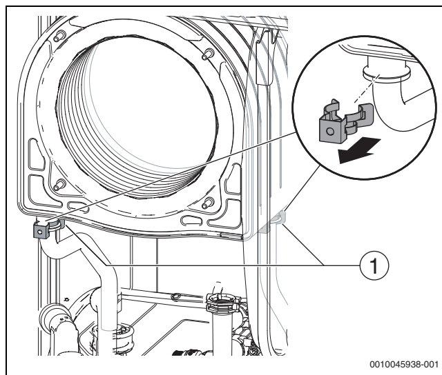
Fig. 103 Smontaggio delle fascette stringitubo
