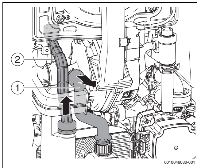
Fig. 117 Scollegamento del flessibile per condensa e del flessibile di collegamento gas
