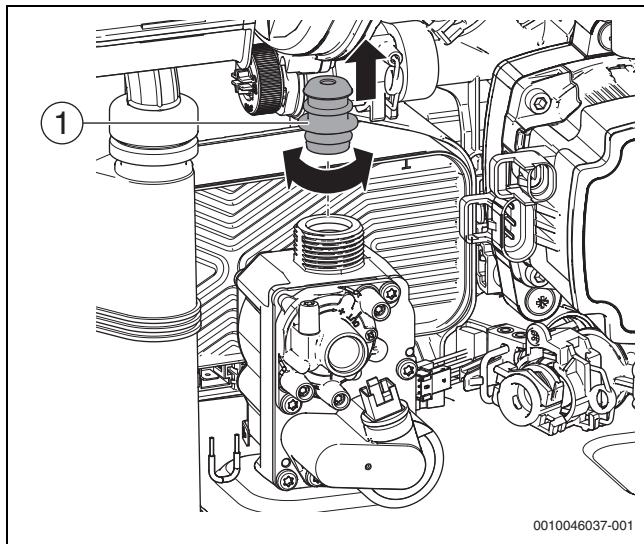
Fig. 123 Smontaggio del diaframma
