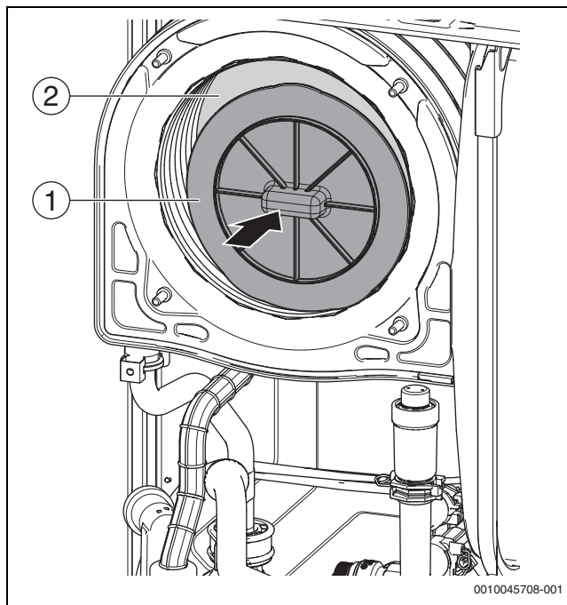
Fig. 49 Protezione dell'isolamento
