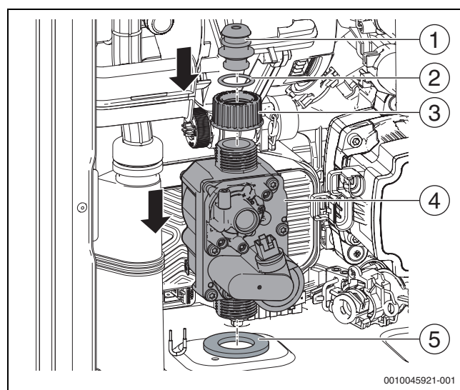
Fig. 95 Montaggio della valvola del gas
