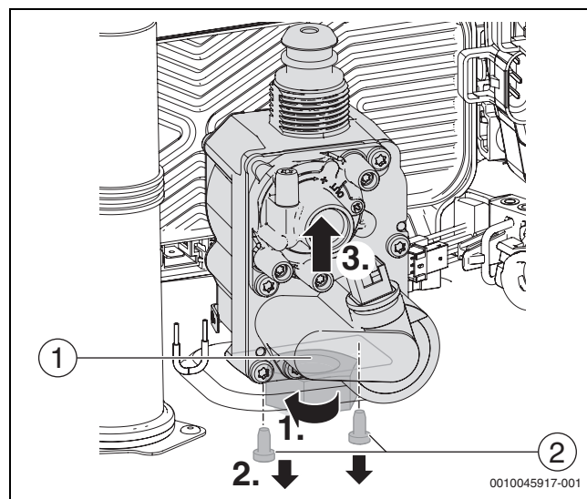
Fig. 94 Smontaggio della valvola del gas
