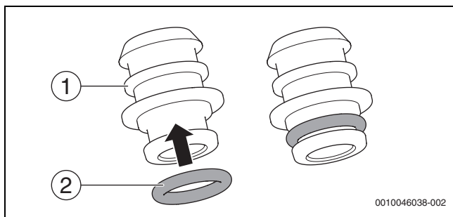
Fig. 124 Applicazione della guarnizione o-ring sul diaframma
