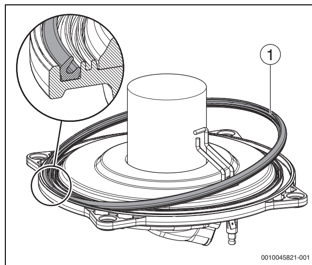
Fig. 71 Sostituzione della guarnizione profilata
