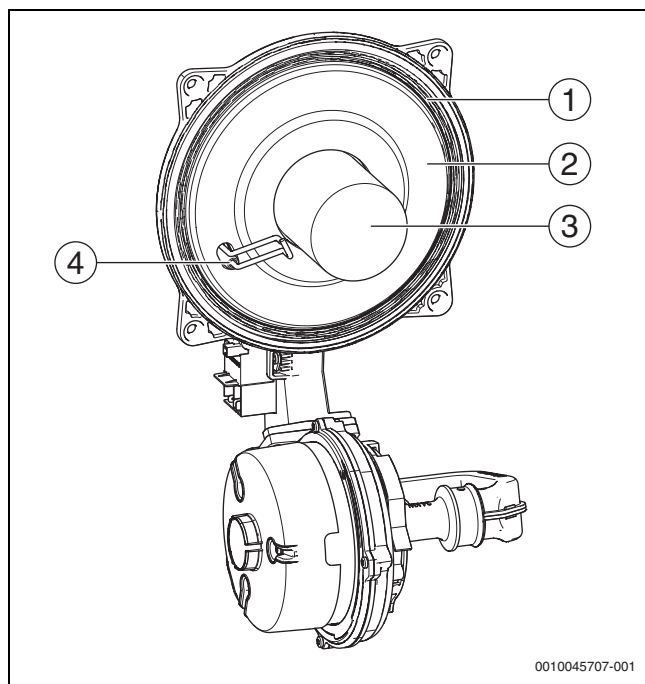
Fig. 54 Sportello bruciatore
