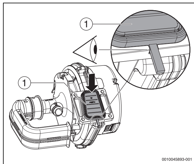
Fig. 86 Posizione della protezione antiriflusso sull'involucro
