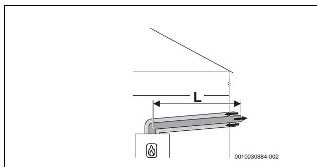
Fig. 7 Condotto di aspirazione aria comburente/evacuazione pdc orizzontale concentrato secondo C_{13x} attraverso la parete esterna
