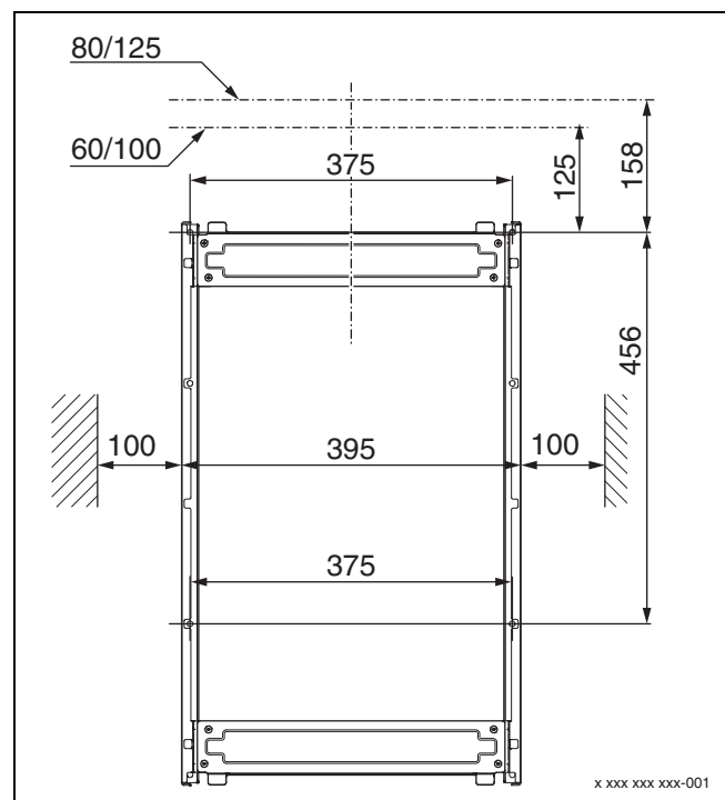
Fig. 3 Dimensioni e distanze minime telaio posteriore (mm)
