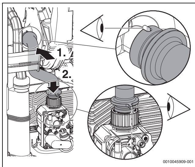
Fig. 90 Montaggio del flessibile di collegamento gas
