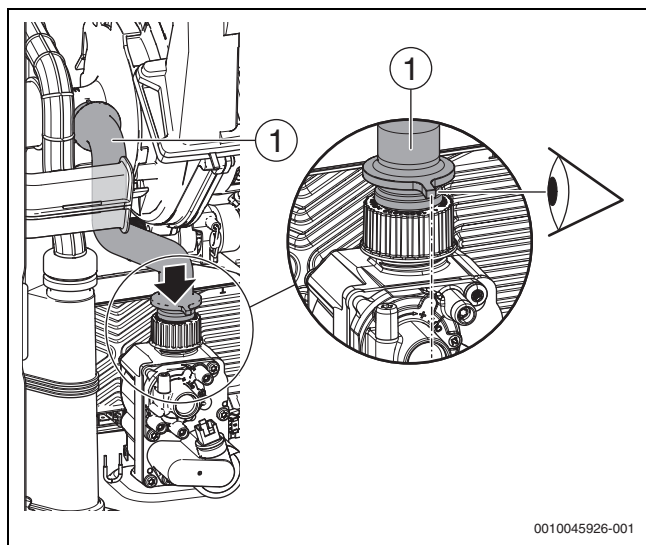
Fig. 97 Montaggio del flessibile di collegamento gas
