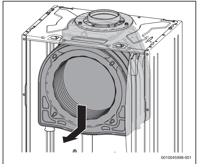
Fig. 106 Estrazione dello scambiatore di calore
