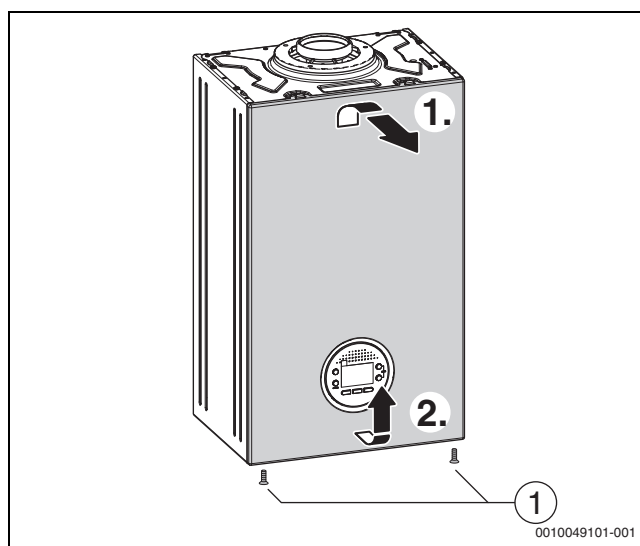
Fig. 43 Rimozione del rivestimento anteriore
