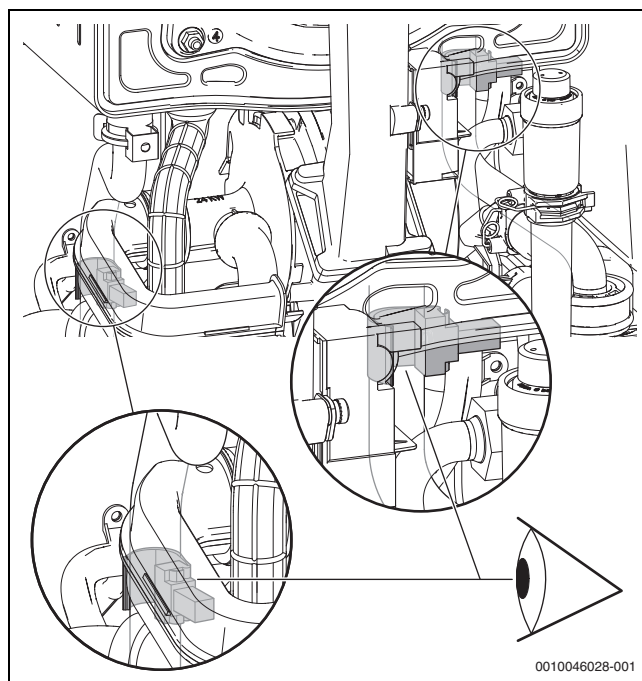
Fig. 58 Posizione sonde NTC
