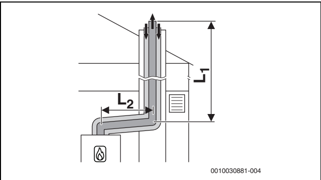
Fig. 9 Condotta di aspirazione aria comburente/evacuazione prodotti della combustione concentrico secondo C 33x nel cavedio
