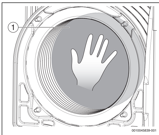
Fig. 77 Posizionamento del disco isolante
