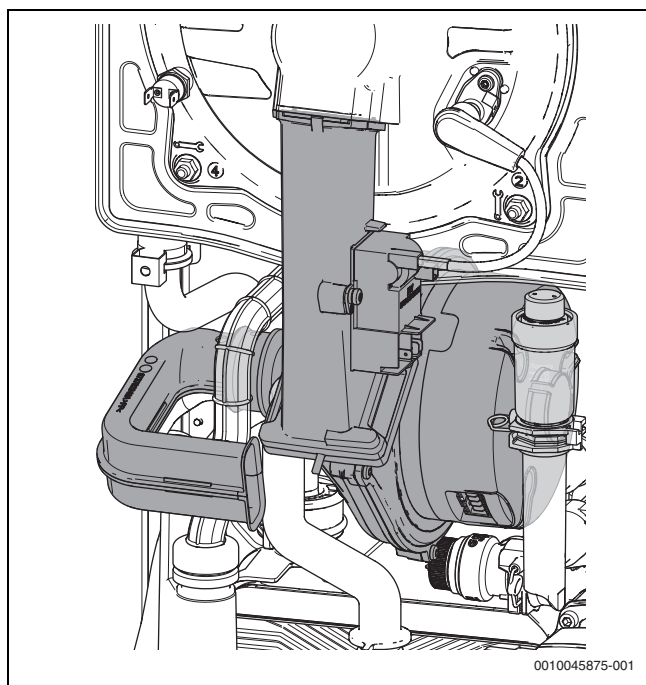
Fig. 81 Smontaggio dei componenti
