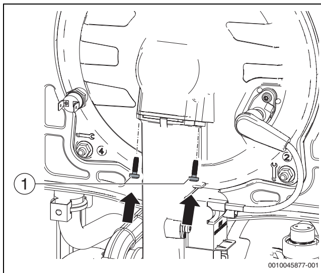
Fig. 121 Montaggio delle viti nello sportello della camera di combustione
