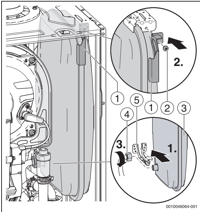
Fig. 139 Montaggio del vaso d'espansione nuovo
