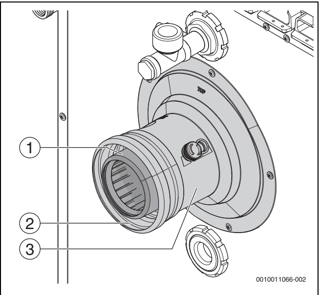
Fig. 19 Montaggio del collegamento di scarico dei gas combusti
