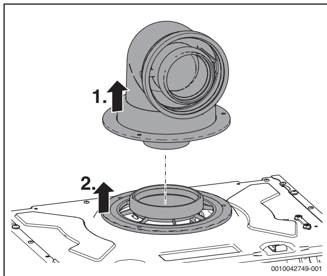
Fig. 150 Smontaggio del set condotto di evacuazione prodotti della combustione
