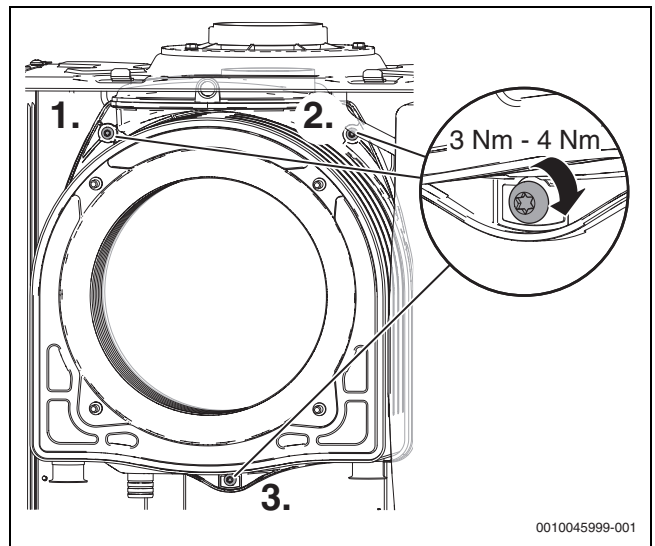
Fig. 107 Montaggio dello scambiatore di calore nuovo
