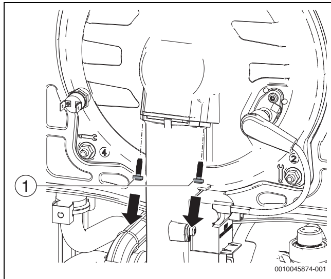
Fig. 127 Smontaggio delle viti
