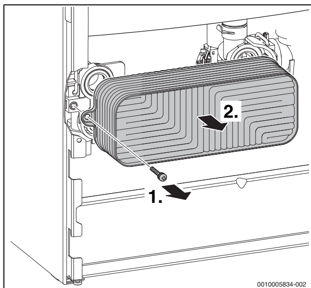
Fig. 144 Smontaggio dello scambiatore di calore a piastre
