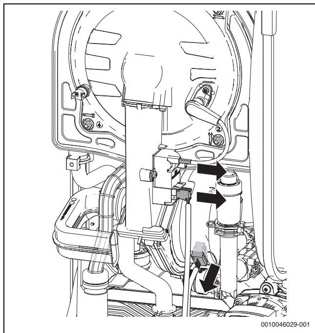
Fig. 116 Scollegamento dei cavi conduttori
