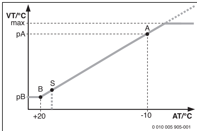
Fig. 158 Curva termocaratteristica
