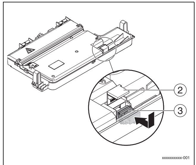
Fig. 141 Inserimento della chiave di codifica
