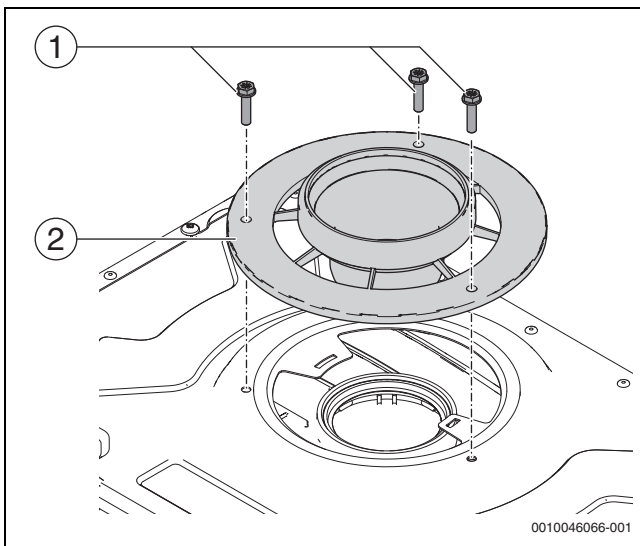
Fig. 64 Montaggio del set condotto di evacuazione prodotti della combustione e dell'adattatore per condotto gas combusti
