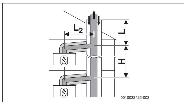
Fig. 22 Collettore scarico gas combusti secondo C (14)3x con sistema di aspirazione aria comburente/evacuazione prodotti della combustione collettivo concentrico e condotto di aspirazione aria comburente/evacuazione prodotti della combustione concentrico nel luogo di posa
