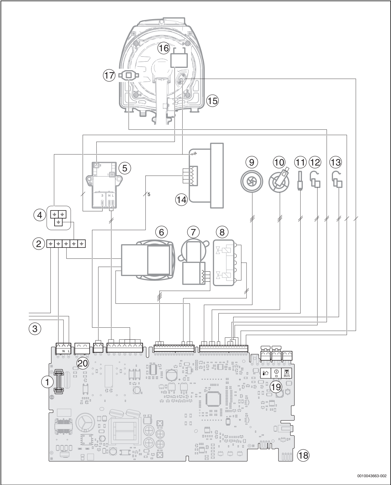
Fig. 157 Cablaggio elettrico
